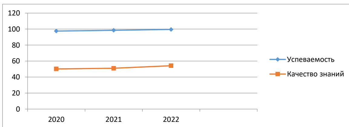
Рисунок 1. Успеваемость и качество знаний (%) за период с 2020 по 2022 г.г.
